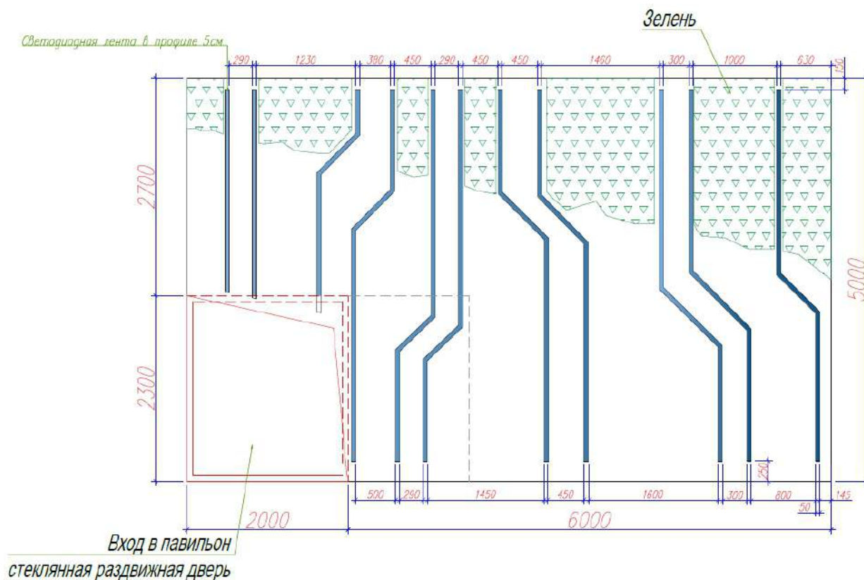
Рис. 17 - Размерный чертеж Центрального модуля (проекция "Вид спереди")
