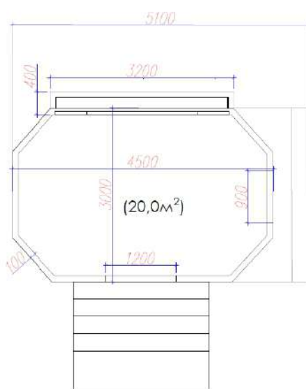
Рис. 14 - Размерный чертеж зоны "Спорт" (проекция "Вид сверху")
