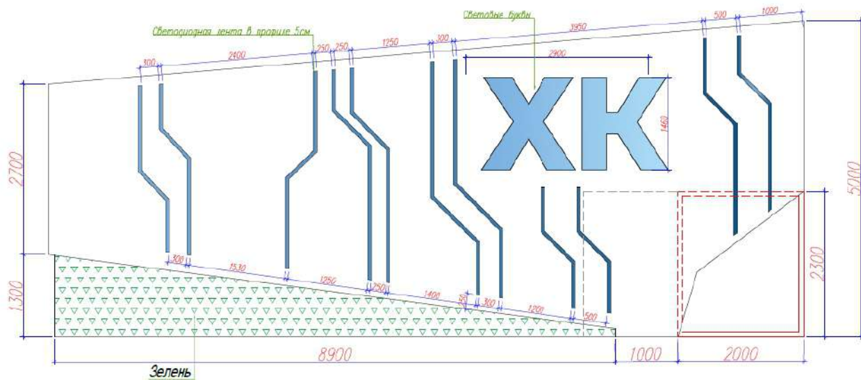
Рис. 16 - Размерный чертеж Центрального модуля (проекция "Вид сбоку")
