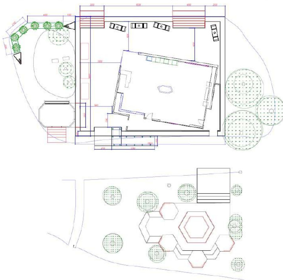
Рис. 12 - Размерный план Павильона края (проекция "Вид сверху")
