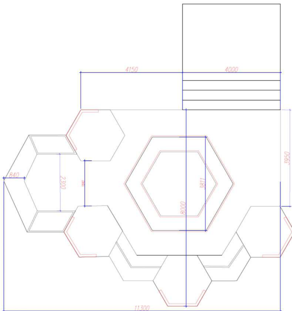
Рис. 13 - Размерный план зоны эко-парк "Технопарк" (проекция "Вид сверху")
