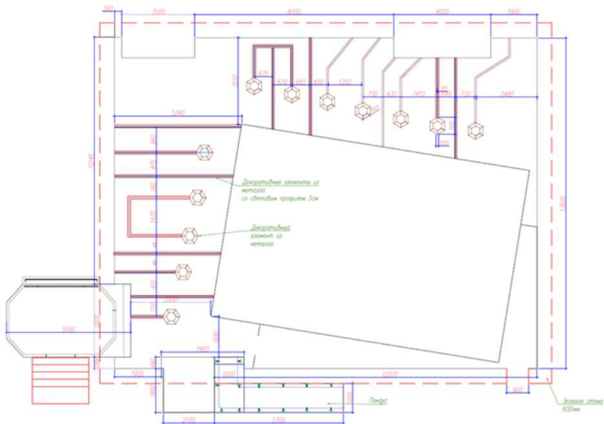
Рис. 15 - Размерный чертеж декоративных световых элементов Павильона края (проекция "Вид сверху")
