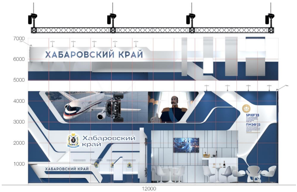
Рис. 8 - Размерный план Выставочного стенда (проекция "Вид сверху")
