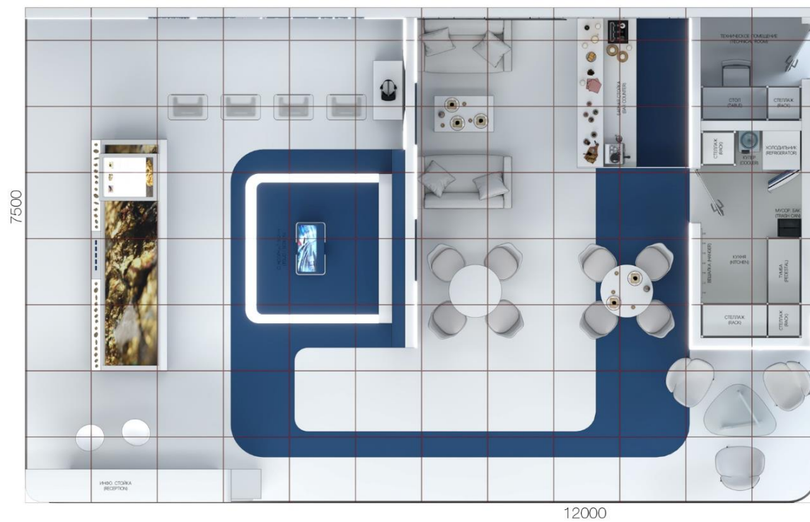
Рис. 9 - Размерный план Выставочного стенда (проекция "Вид сверху")
