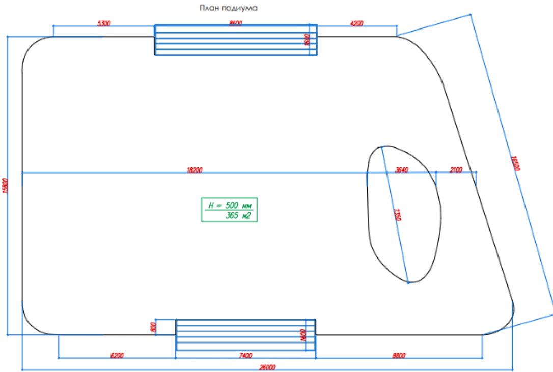
Рис. 25 - Размерный план подиума основного здания (проекция "Вид спереди")
