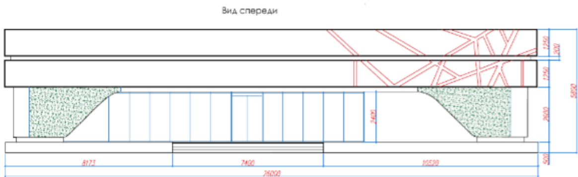
Рис. 22 - Размерный чертеж фасада основного здания (проекция "Вид спереди")
