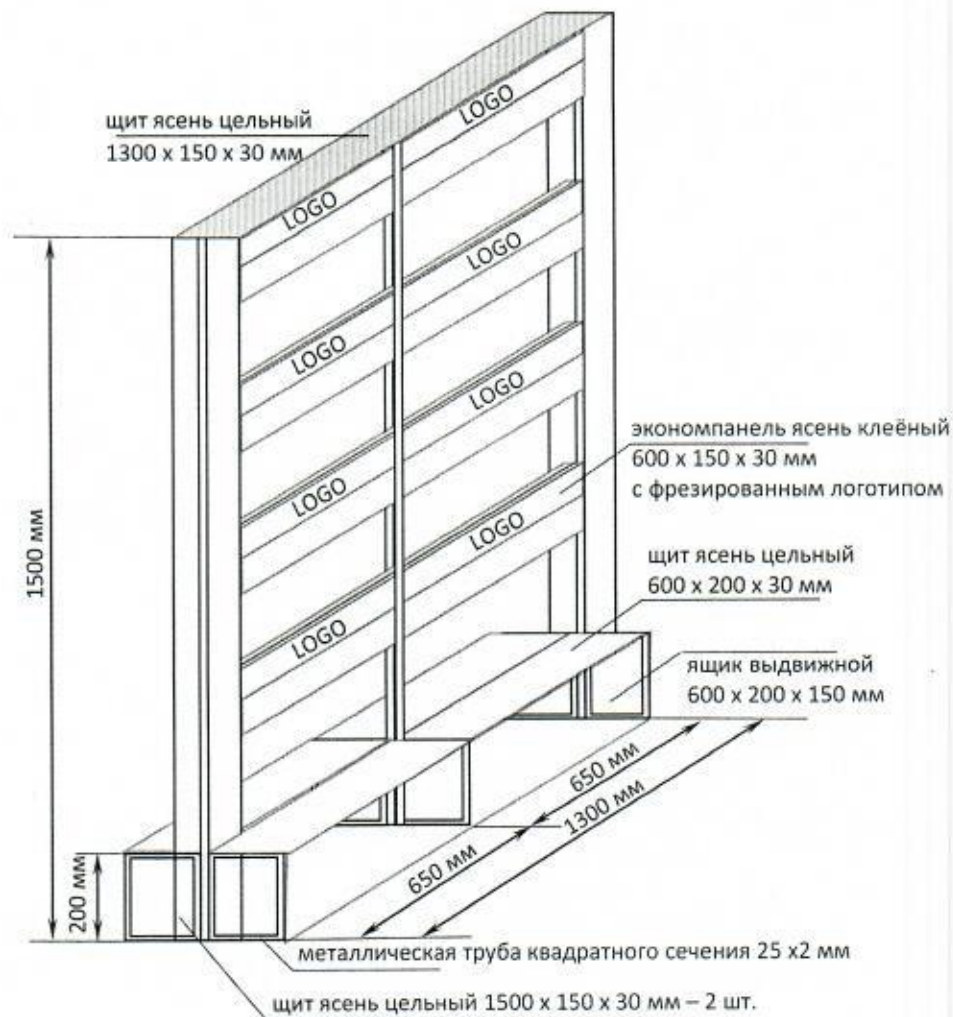
Эскиз демонстрационного стенда
