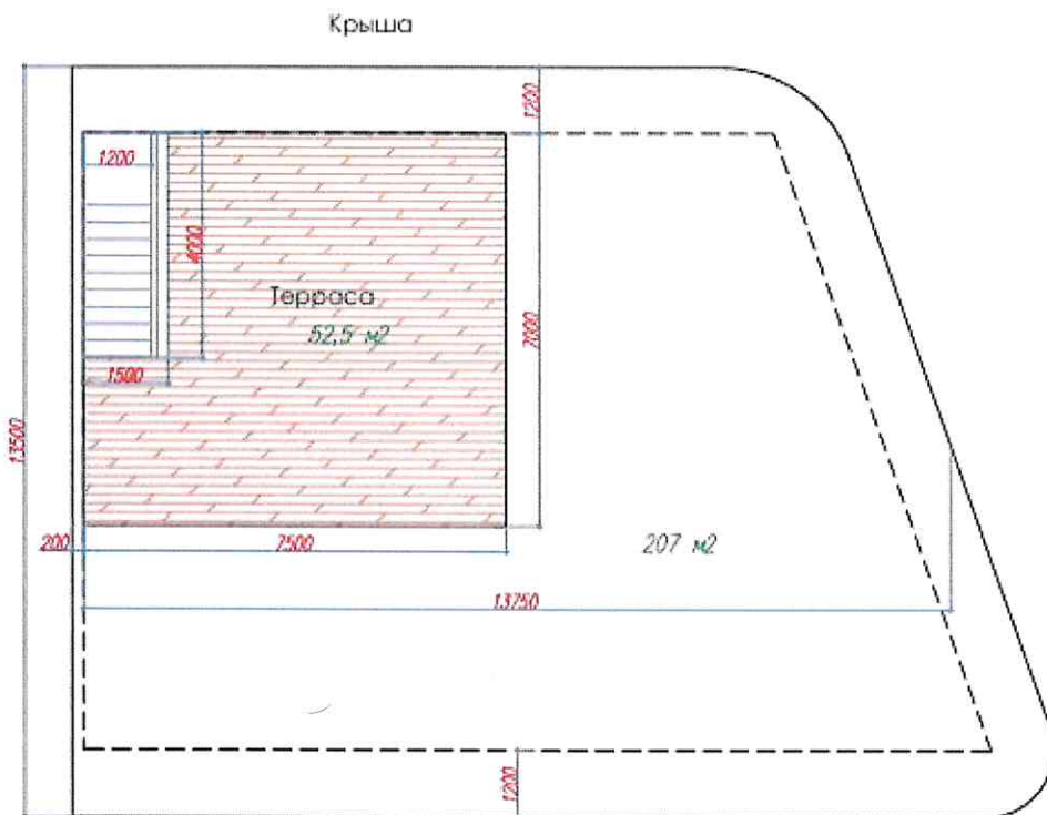
Рис. 28 – Размерный чертеж крыши Павильона края (проекция "Вид сверху")
