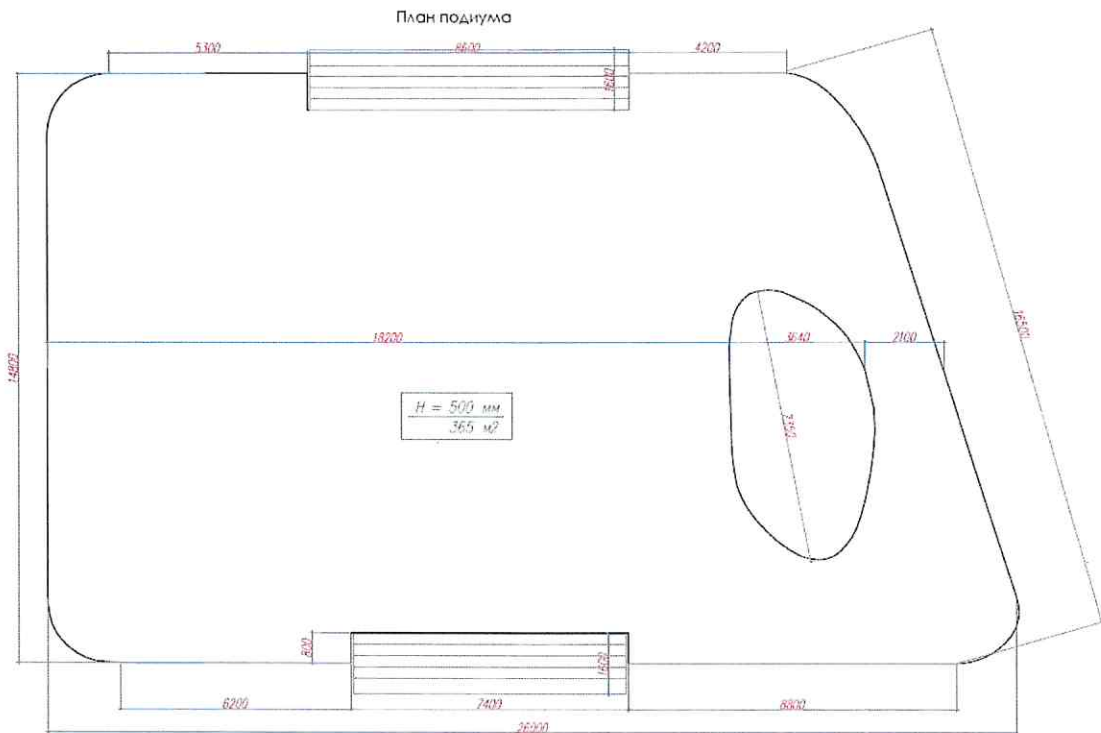
Рис. 27 – Размерный план подиума Павильона края (проекция "Вид спереди")
